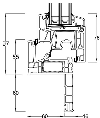
Montante fisso standard - Anta standard 76372 - 76271
