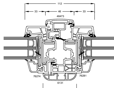
Maniglia centrale 6131 - 76274 - 76281
