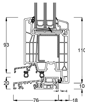
Soglia bassa - Anta intermedia A076 - A062 - 76272
