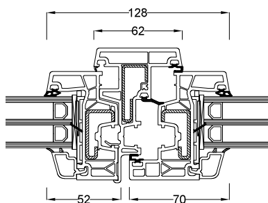
Anta ribassata - Montante mobile stretto 76270 - 76471
