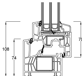
Telaio normale - Anta ribassata 76171 - 76270
