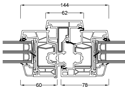
Anta standard - Montante mobile stretto 76271 - 76471
