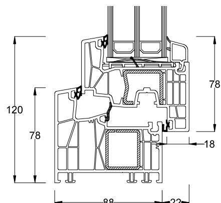
Telaio normale-Anta standard 88171 - 88271
